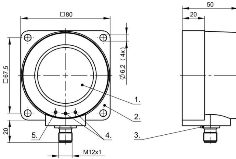
1) 有效面 2) 外壳 3) 盖子 4) 功能显示, 黄色 5) 回波显示, 绿色
